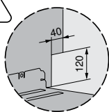
Piastra di supporto per installazione a colonna
